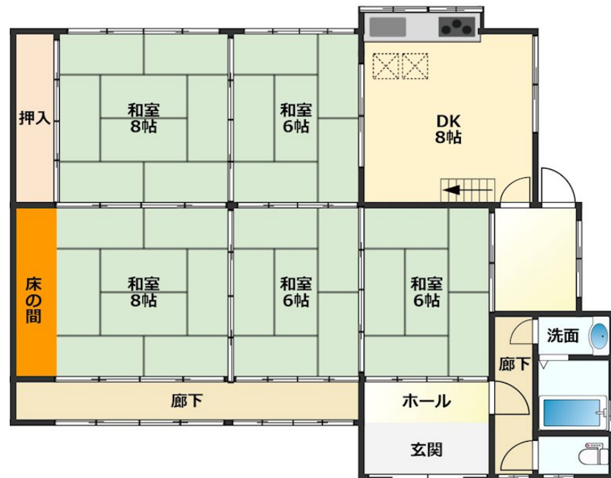
【間取り図】
